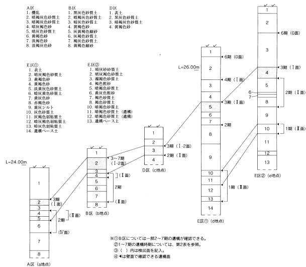
第4図 基本土層柱状図
