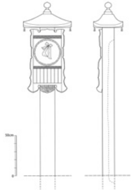
笠塔婆想定復元図
