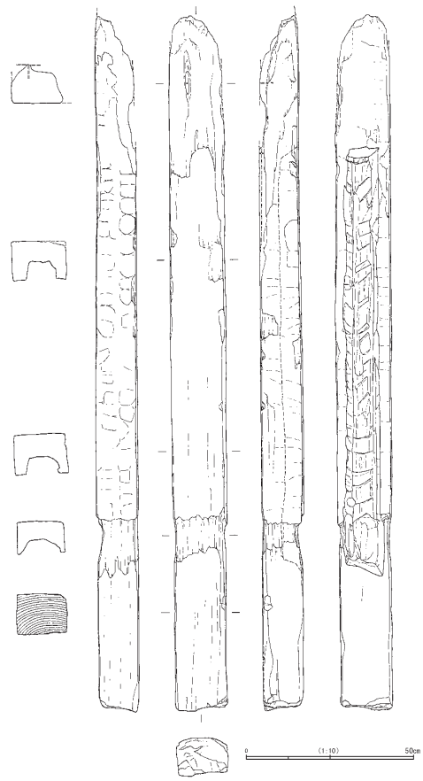
木製板碑部分名称と実測図 (S= 1 / 10)
