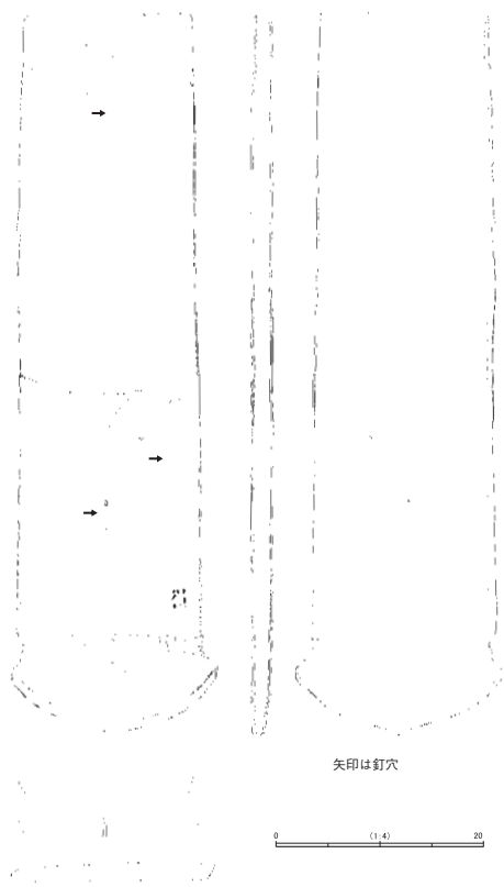
木製板碑部分名称と実測図 (S= 1 / 10)
