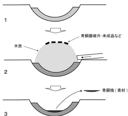
SI04火窪炉の築造・操業概念図 (鄭宗編作成)
