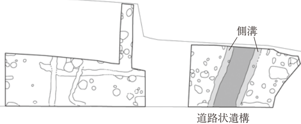
第3面遺構平面図 (S=1/600)
