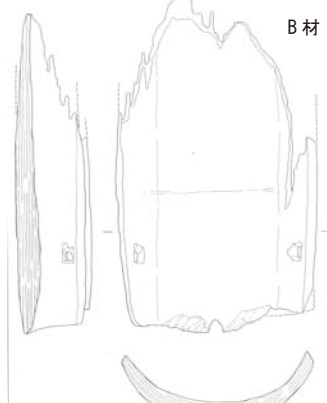
額見町遺跡・準構造船材（船底部）（S=1/40）
