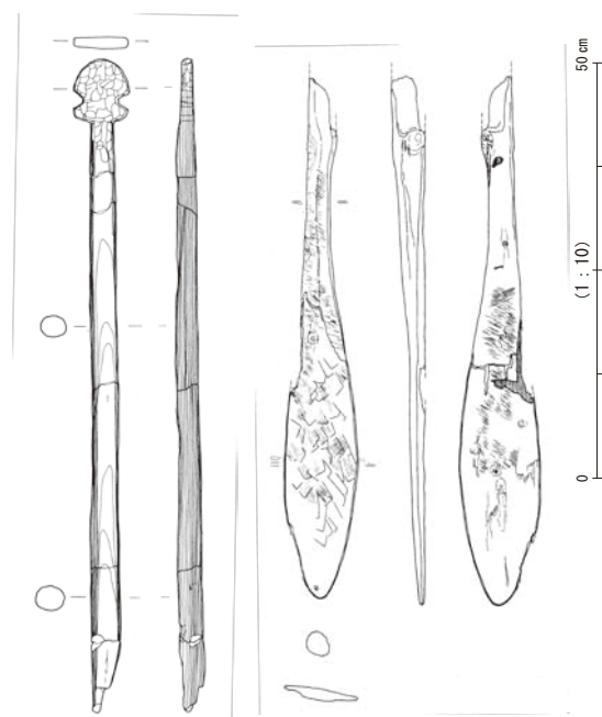
真脇遺跡・櫓 (S=1/10) 三引遺跡・櫓 (S=1/10)
