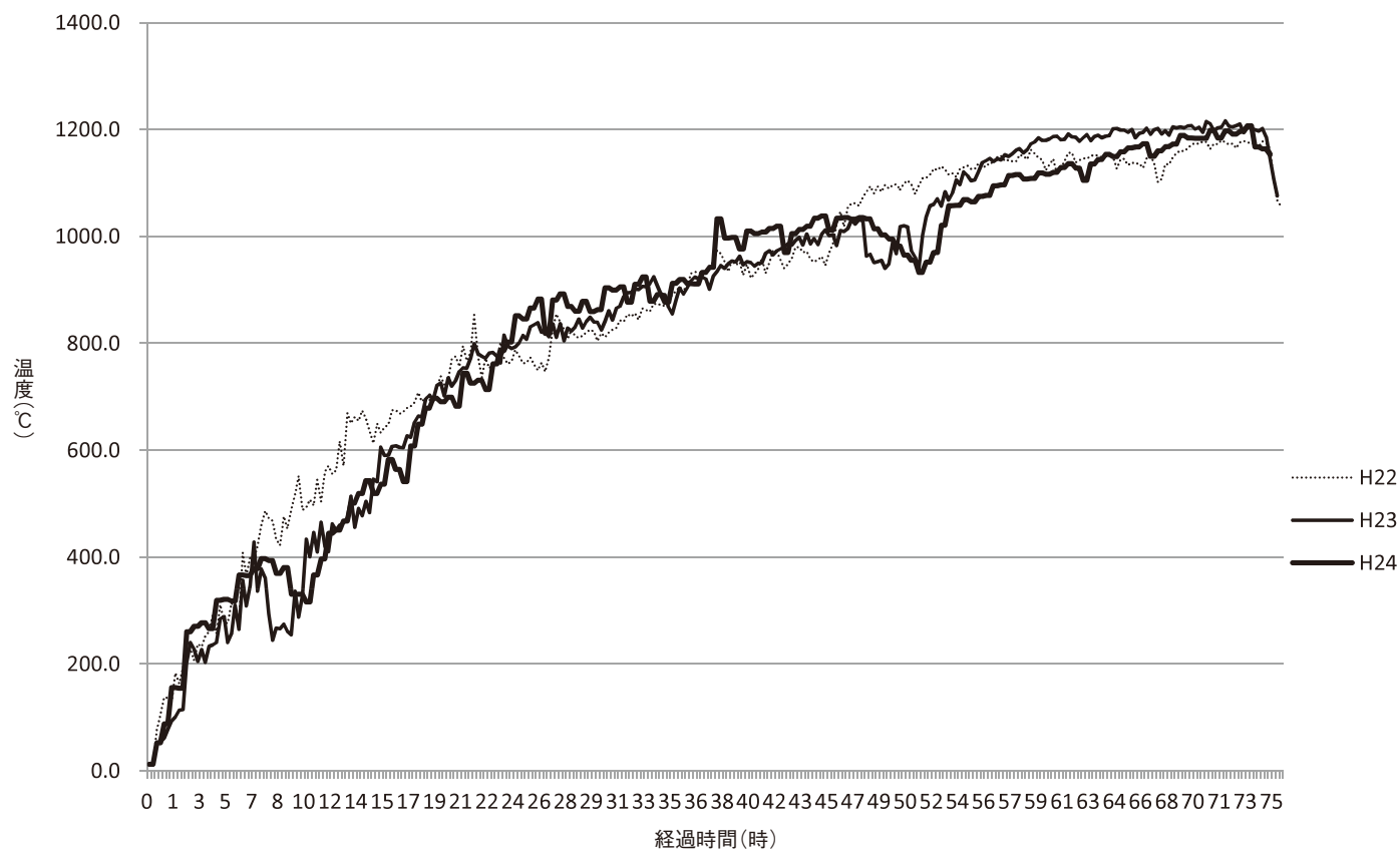
第1図 窯内温度の推移（測点3）
