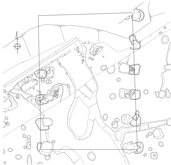
SB205 遺構図 (S=1/150)
