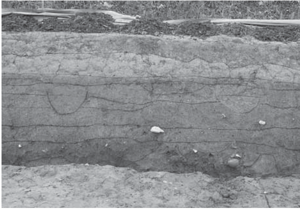
土層断面
