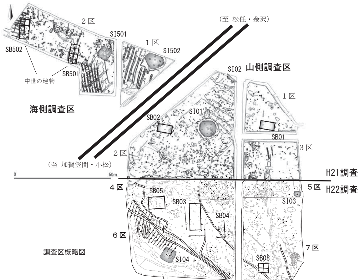
調査区概略図 (平成 21・22 年度調査)
