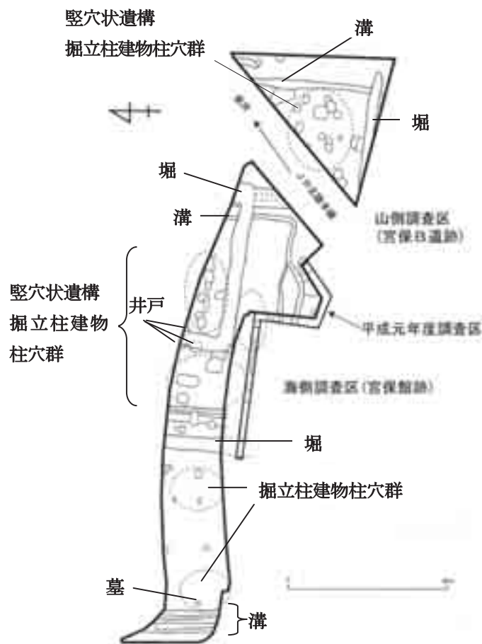
主要遺構配置図 (S=1/2,000)
