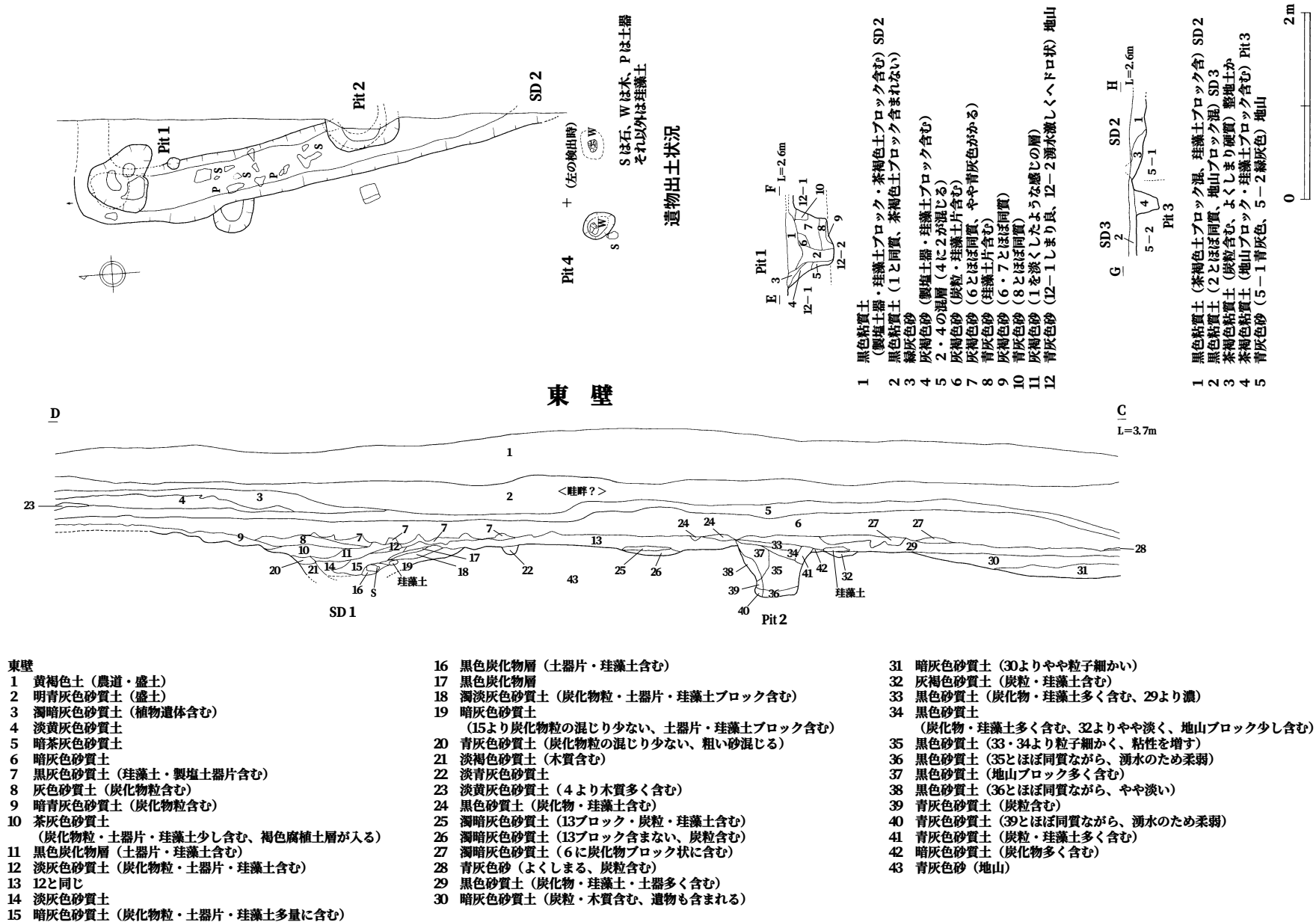
第4図 遺構実測図2 (S=1/60)
